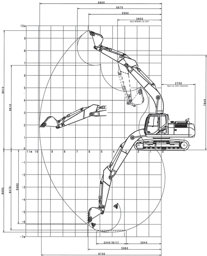
ALCANCE DE EXCAVACIÓN CON BRAZO DE 2,94 M (9' 7,8")
