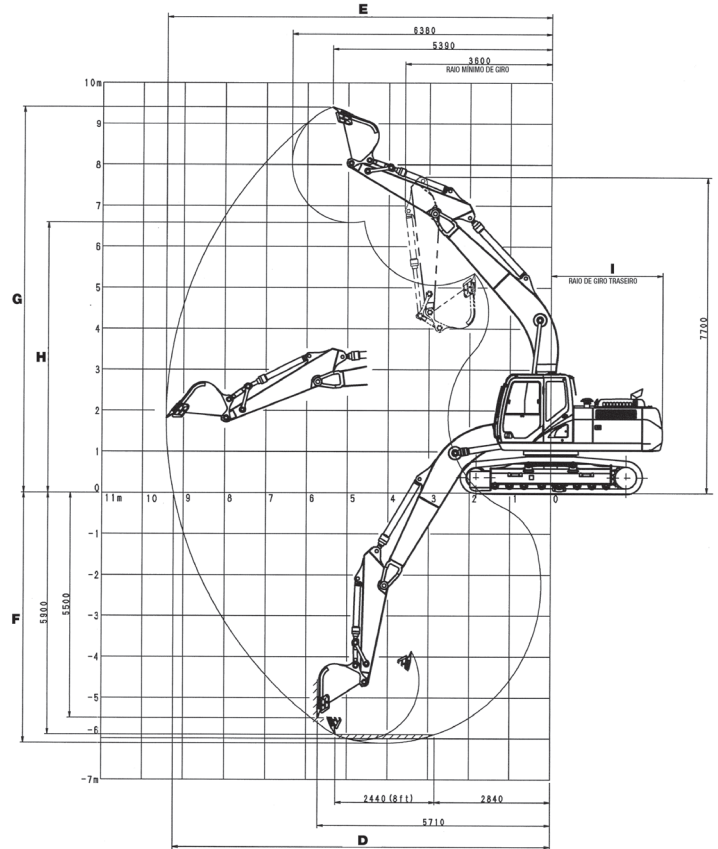
ALCANCE DE EXCAVACIÓN CON BRAZO DE 2,40 M (7' 10,5")
