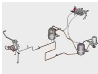
Kit de freio pneumático
