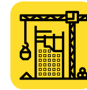
Общестроительные работы
